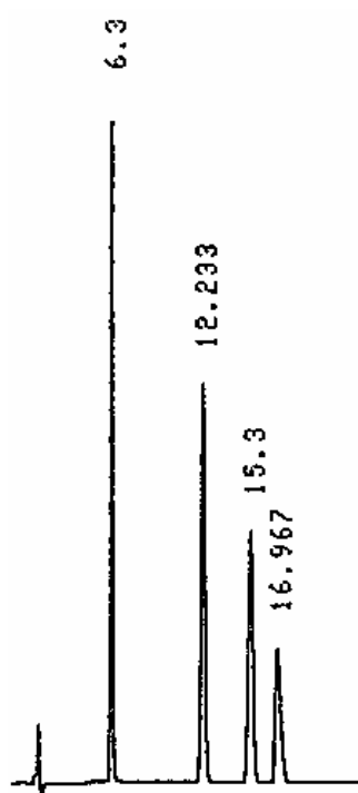
SUMIPAX ODS C-217(5 μm)
